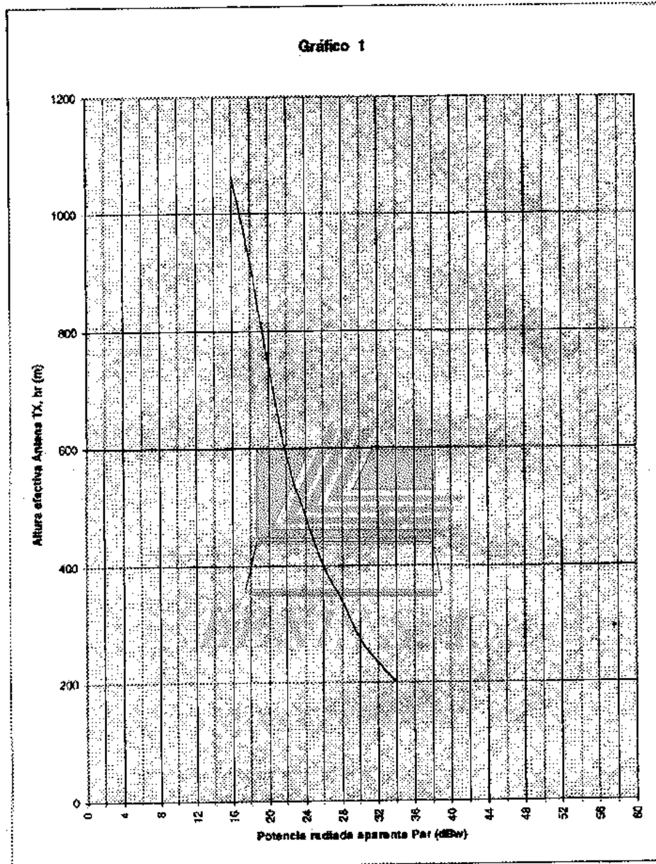
CARACTERÍSTICAS DE ALTURA EFECTIVA DE LA ANTENA TRANSMISORA Y POTENCIA RADIADA APARENTE PARA UNA ZONA DE SERVICIO
